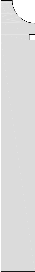
BA 6011LH 3/4 X 6
