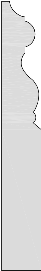
BA 4625LH 11/16 X 4-5/8
