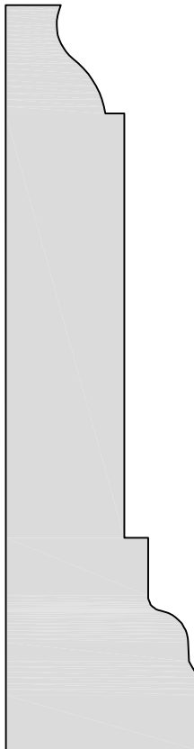
BA 4313LH 1-1/8 X 4-5/16
