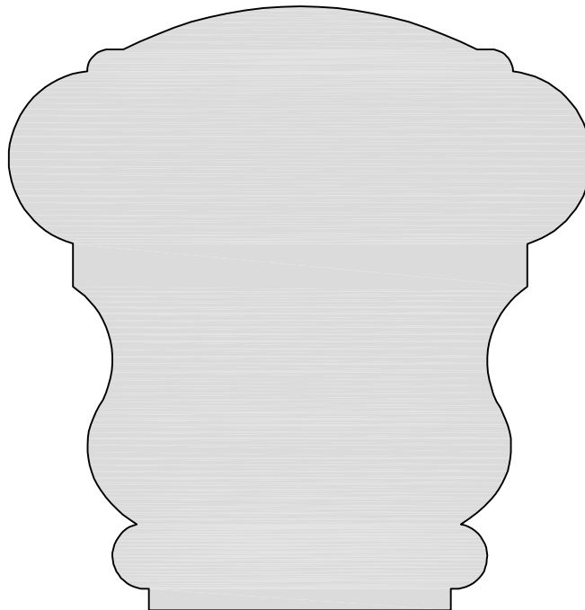
HR 3375 3-1/2 x 3-3/8
